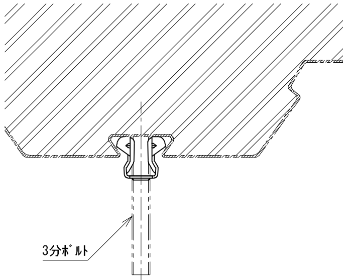
使用状態参考図(1/2)
