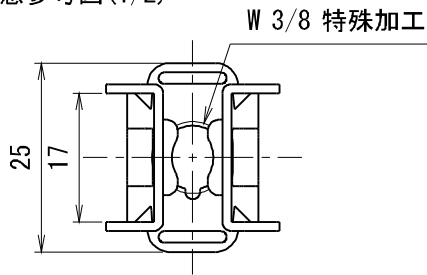
使用状態参考図(1/2)
